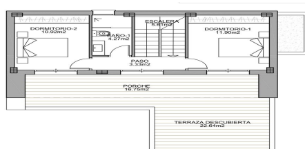
PLANTA PRIMERA
