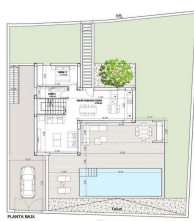
O3. Planta Baja
